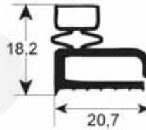
9106
