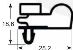
N° profil 9010
