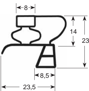
N° profil 9783
