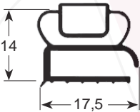
N° profil 9207
